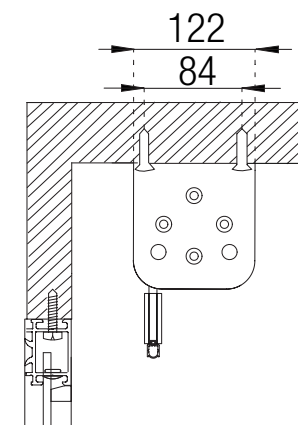
Livorno 122 attacco a soffitto Livorno 122 ceiling mounting
