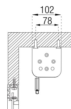
Livorno 102 attacco a soffitto Livorno 102 ceiling mounting
