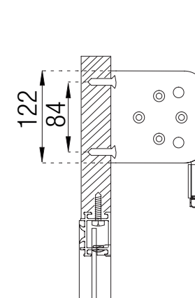
Livorno 122 attacco frontale Livorno 122 wall mounting
