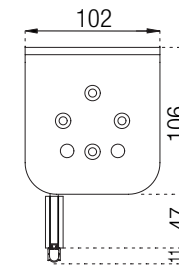
Livorno con supporti 102x106 Livorno with 102x106 brackets
