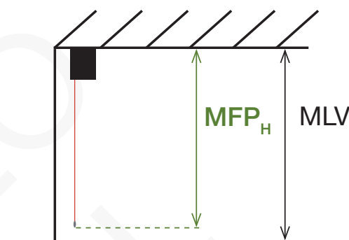
INSTALLAZIONE A SOFFITTO CEILING MOUNTING
