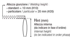
TASCA SALDATA SENZA CHIUSURA ANGOLARE SALDATA WELDED POCKET WITHOUT WELDED ANGULAR ENDING
